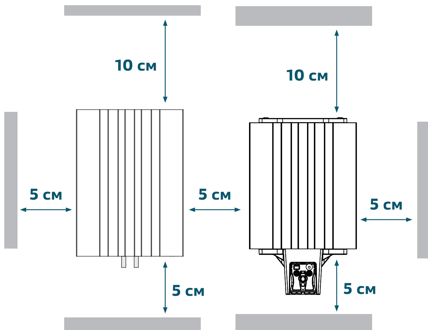
Рис. 1. Минимальные рекомендованные отступы для конвекционных нагревателей SILART
